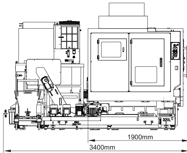
左视图
