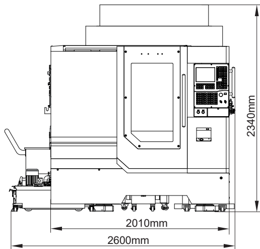
前视图
